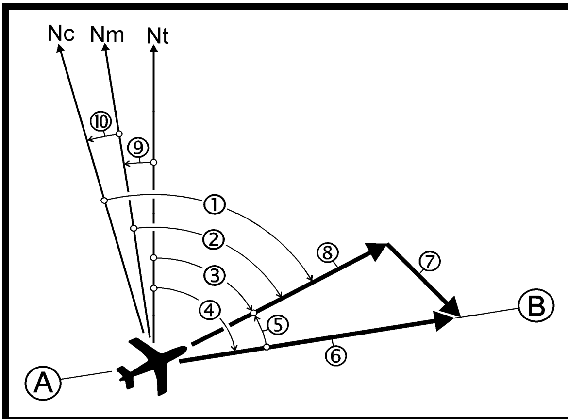
Priloga 12: Trikotnik vetra
