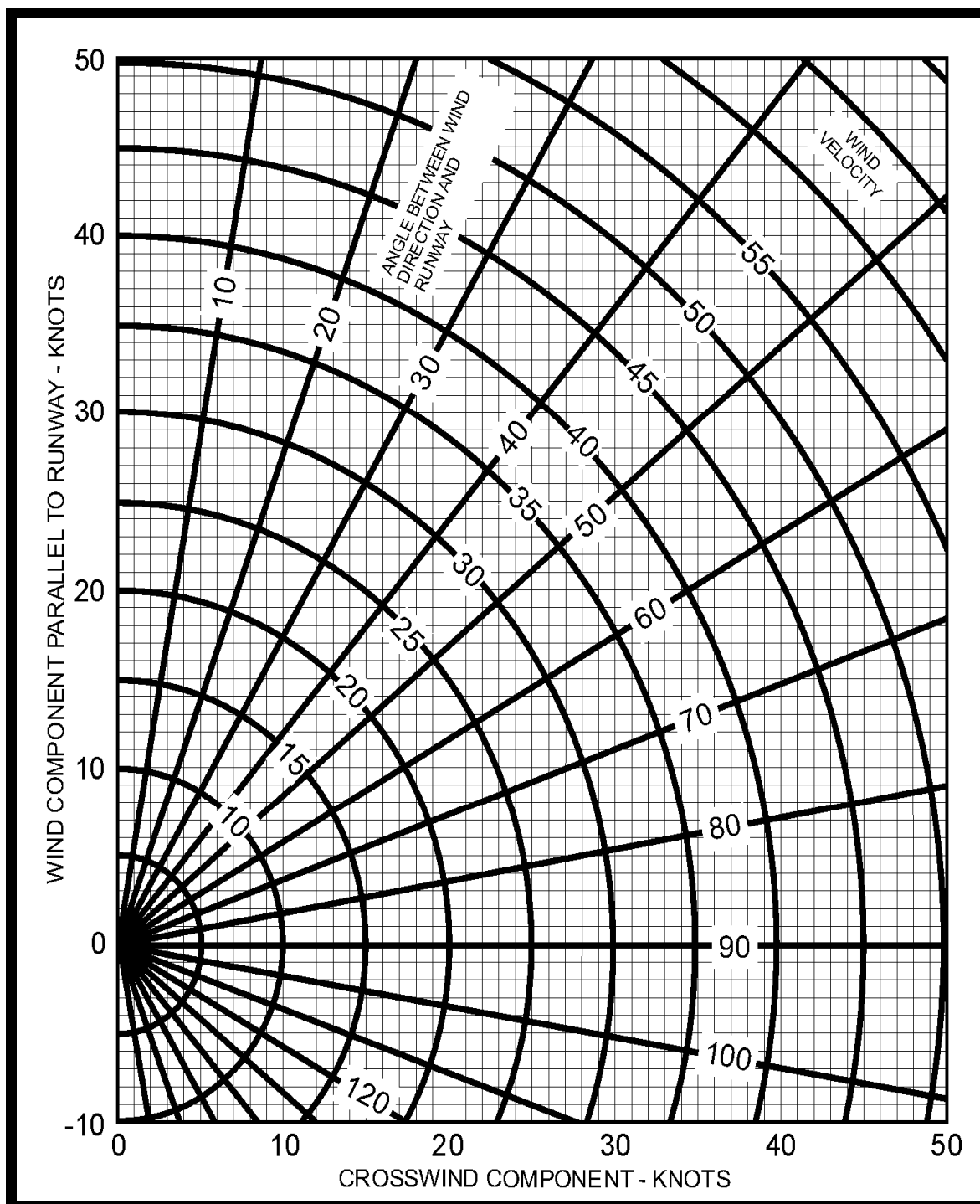
Priloga 14: Grafikon za določanje komponent vetra
