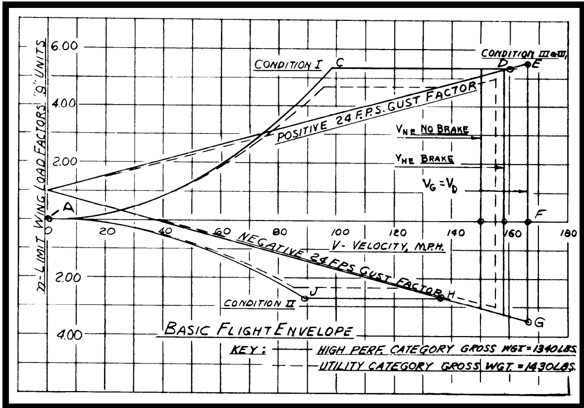
Priloga 4: Manevrska ovojnica jadralnega letala
