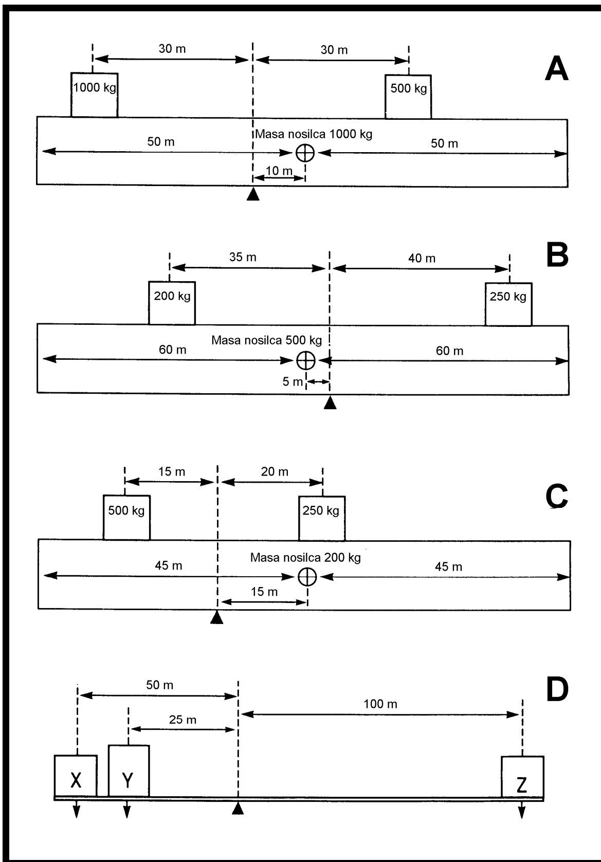
Priloga 6: Ravnotežje vzvoda
