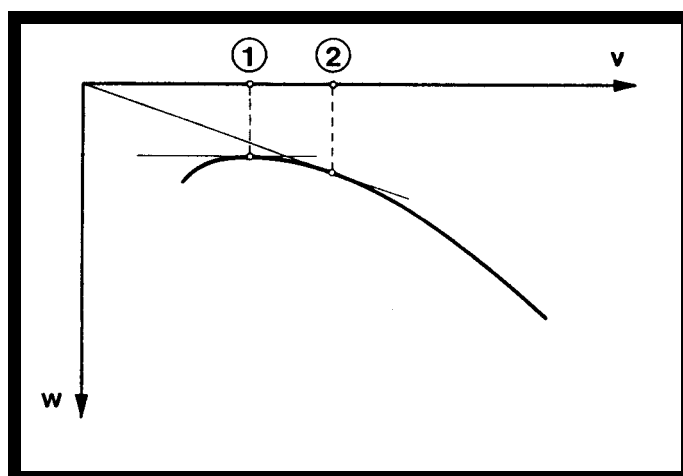
Priloga 9: Značilni točki na hitrostni polari
