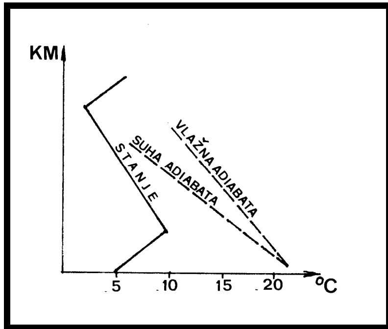
Priloga 15: Emagram
