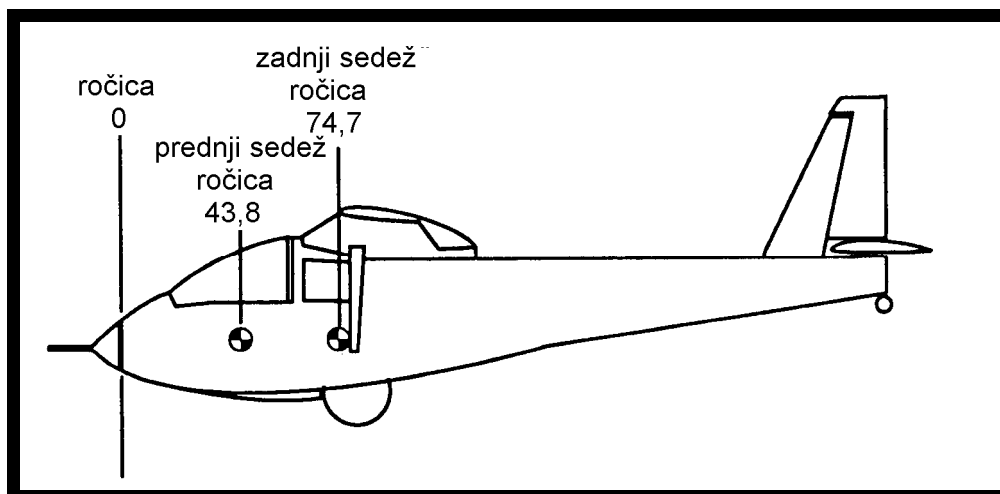
Priloga 7: Uravnoteženje jadralnega letala
