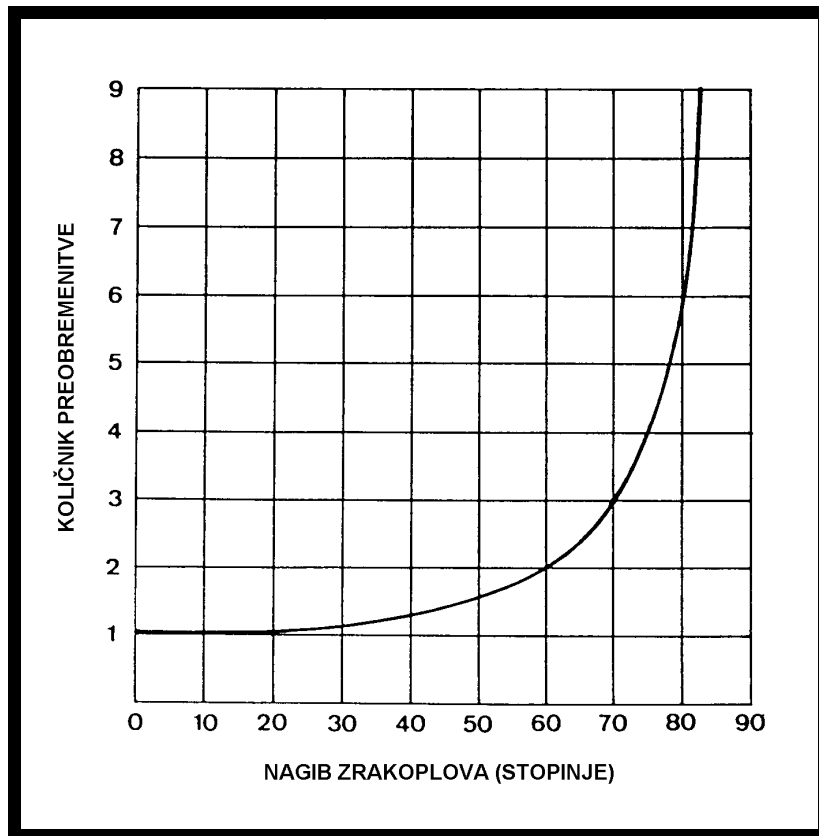
Priloga 5: Odvisnost količnika preobremenitve od nagiba
