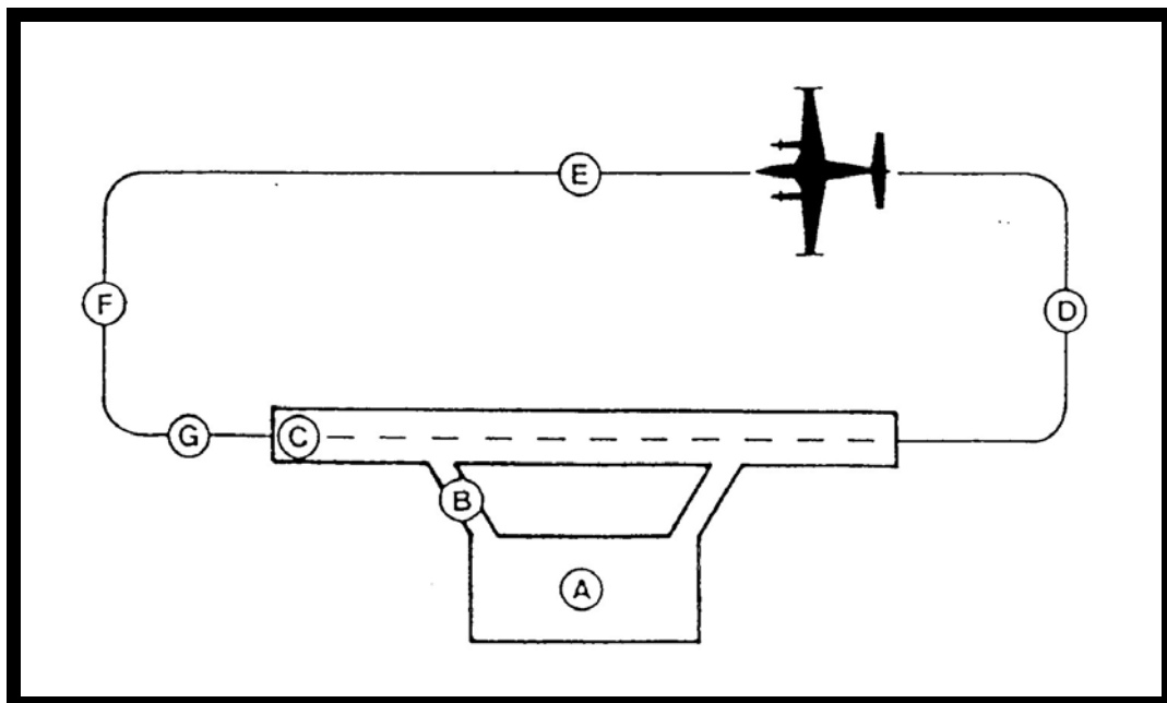
Priloga 16: Letališki krog
