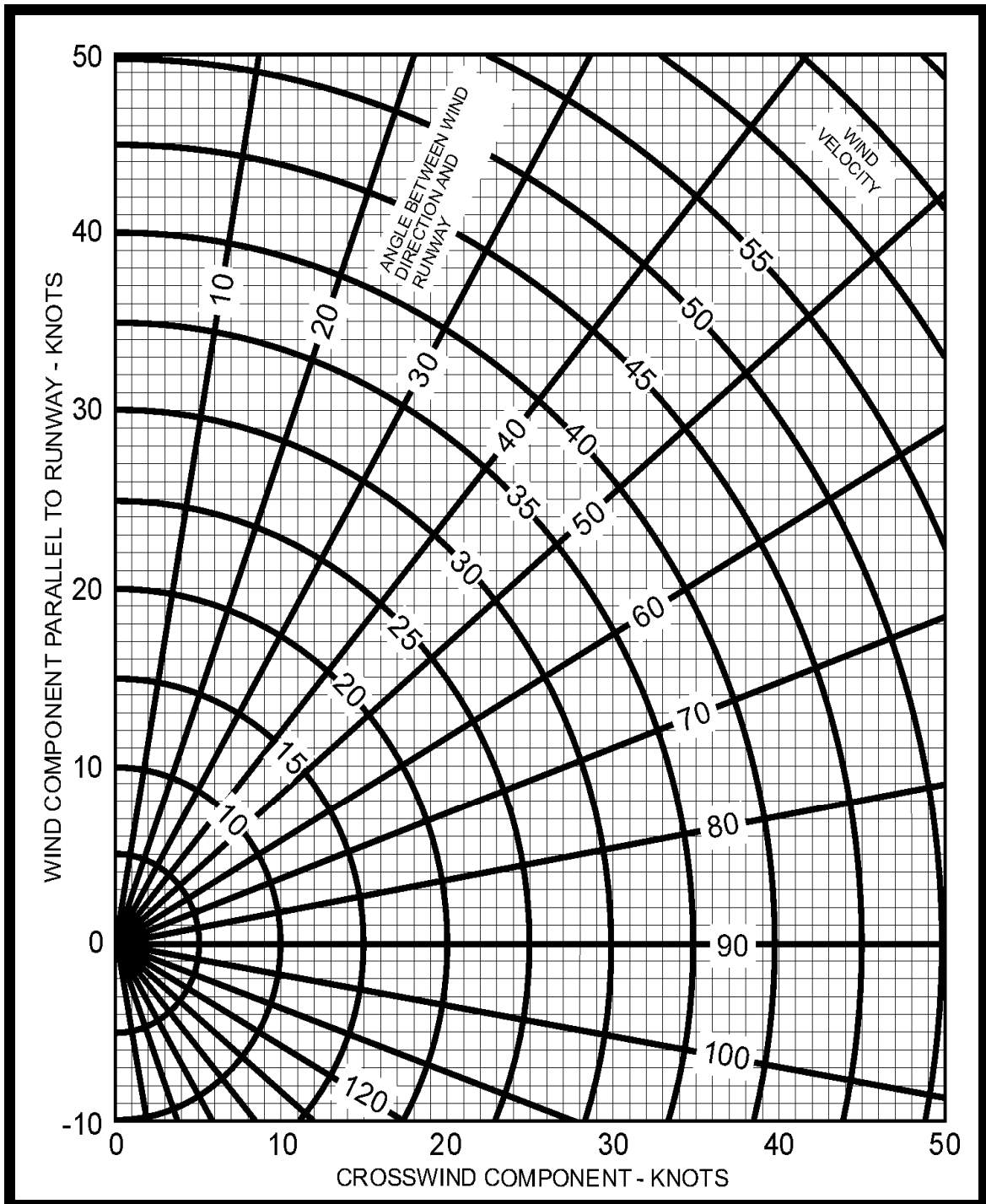
Priloga 9: Grafikon za določanje komponent vetra
