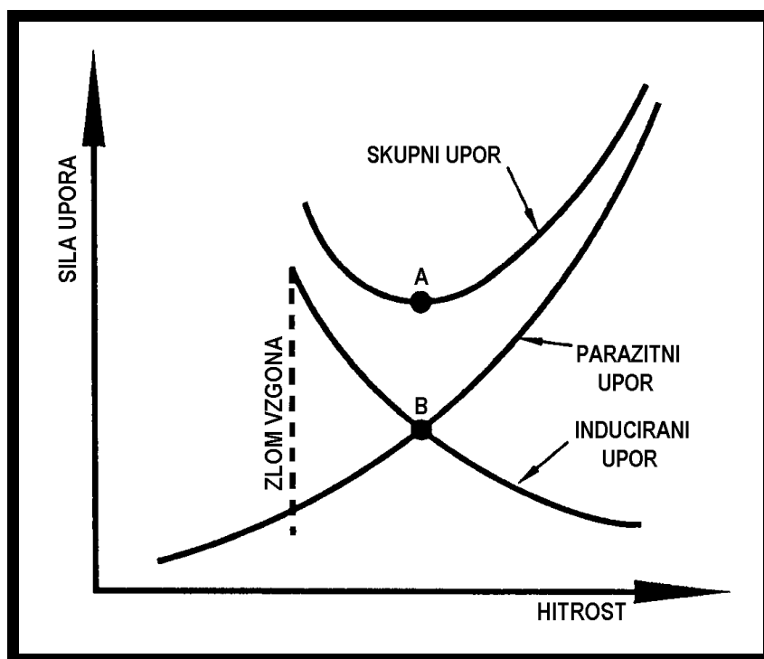
Priloga 2: Sila upora v odvisnosti od hitrosti
