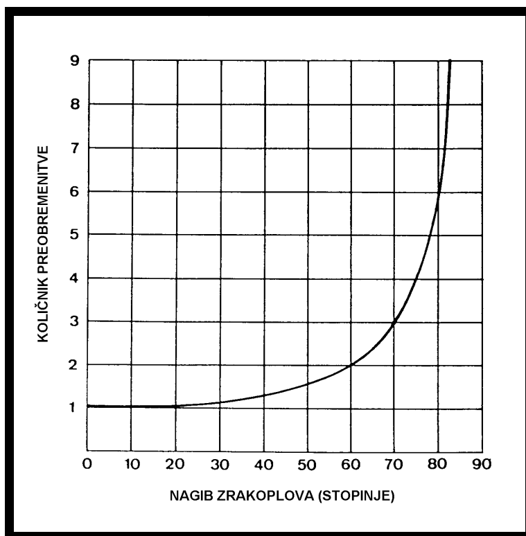
Priloga 4: Odvisnost količnika preobremenitve od nagiba
