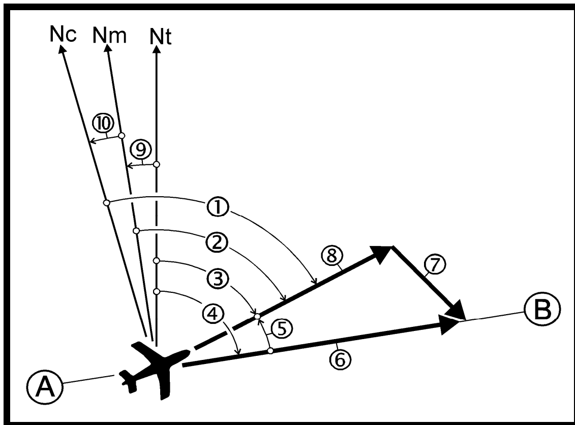
Priloga 7: Trikotnik vetra
