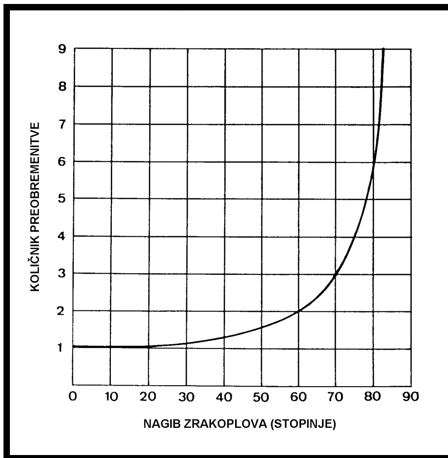
Priloga 4: Odvisnost količnika preobremenitve od nagiba
