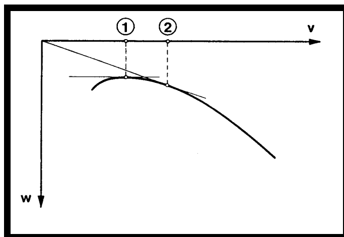
Priloga 10: Značilni točki na hitrostni polari
