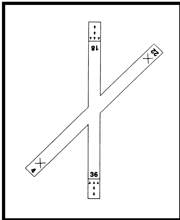
Priloga 10: Označevanje stez
