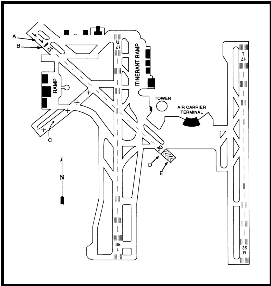
Priloga 9: Oznake na letališču
