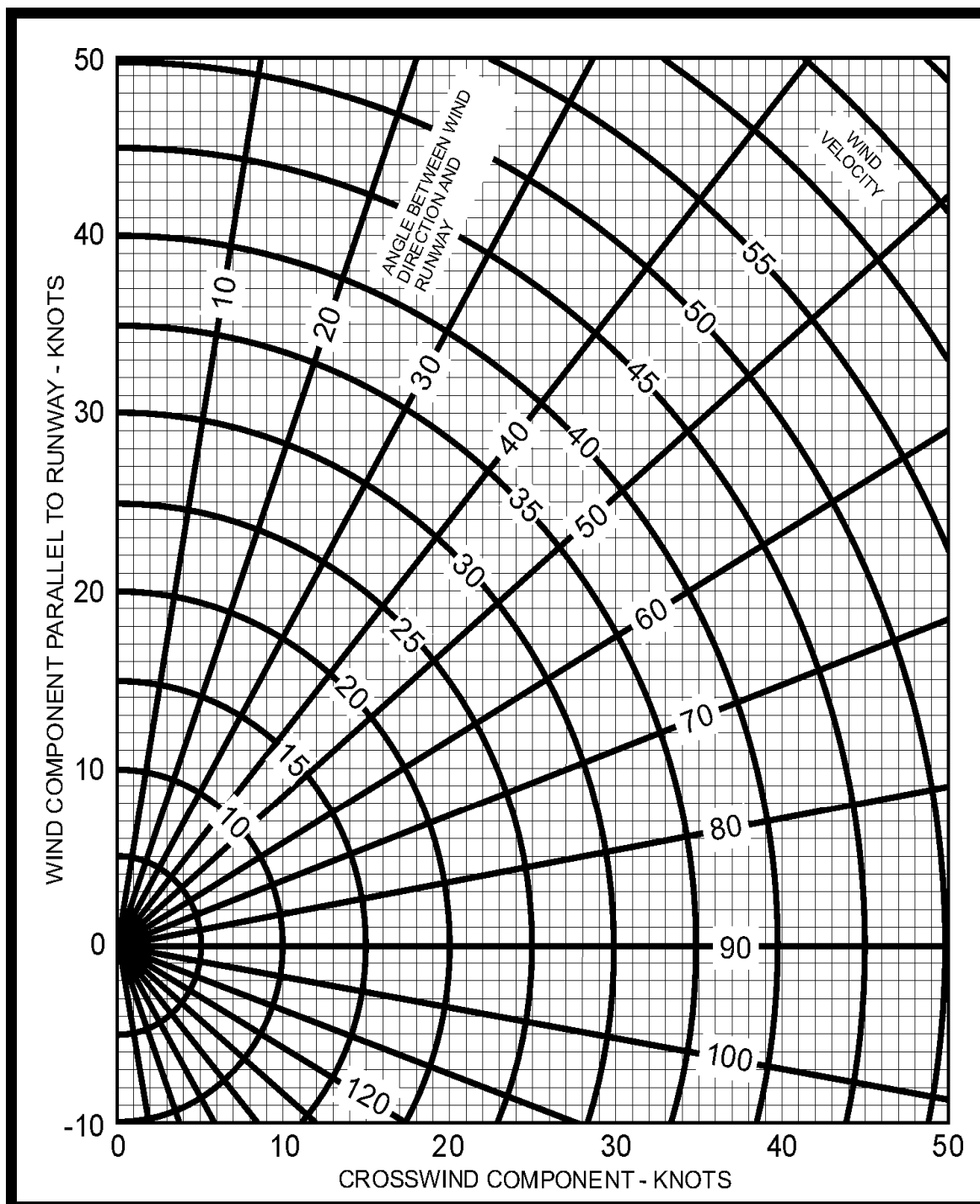
Priloga 7: Grafikon za določanje komponent vetra
